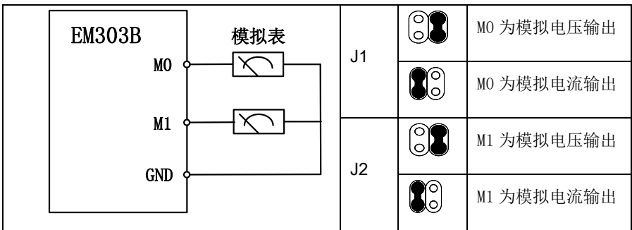
图 3-18 模拟输出端子配线
