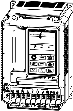
图 2-4 键盘拆卸图示
