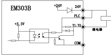
图 3-17 (a) 多功能输出端子用内部电源接线方式
