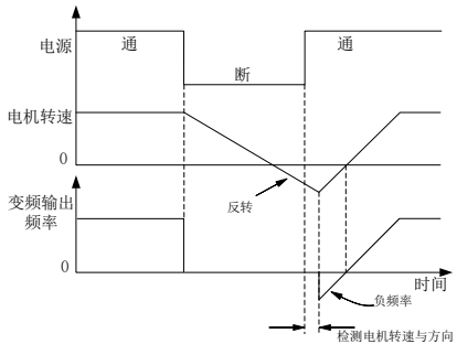
图 7-5 转速追踪启动
