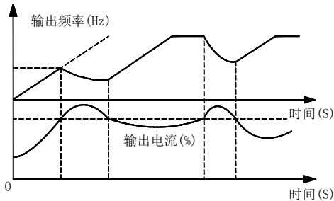
图 7-33 过流失速动作过程
