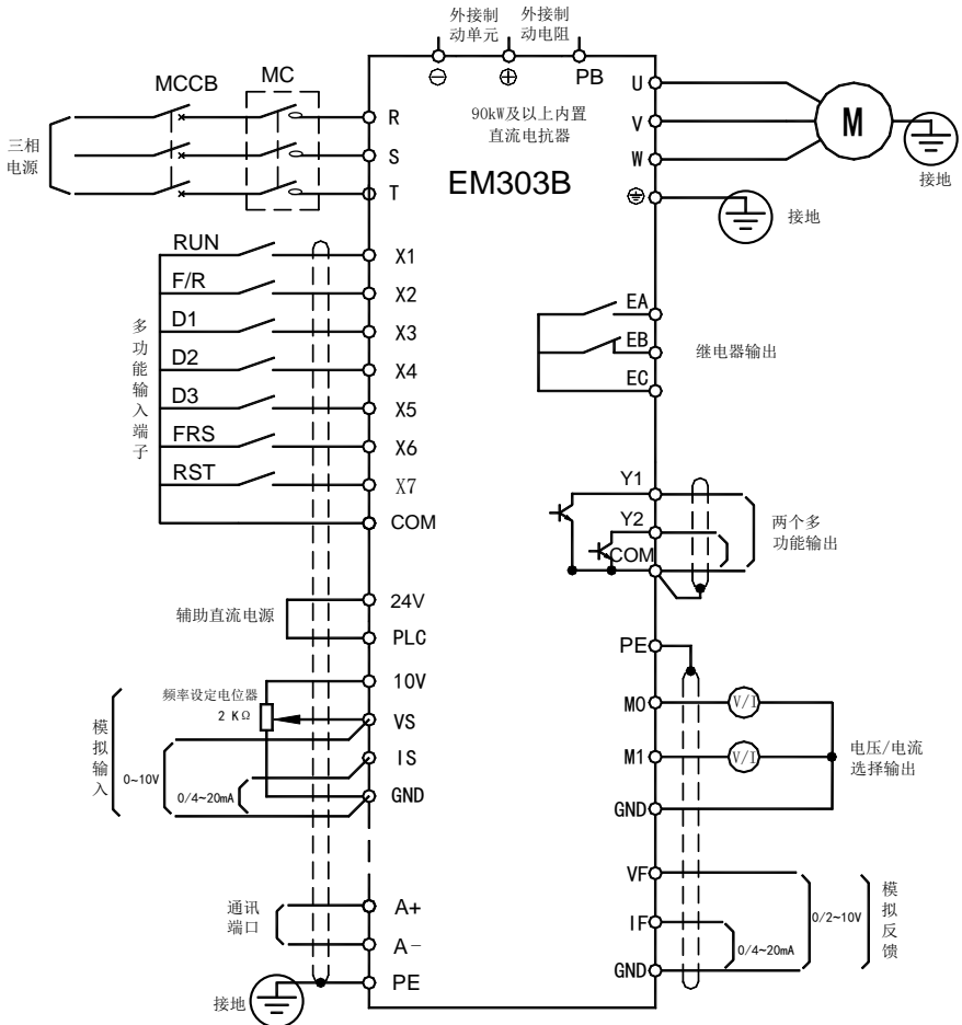
图 3-21 控制回路端子连接图
