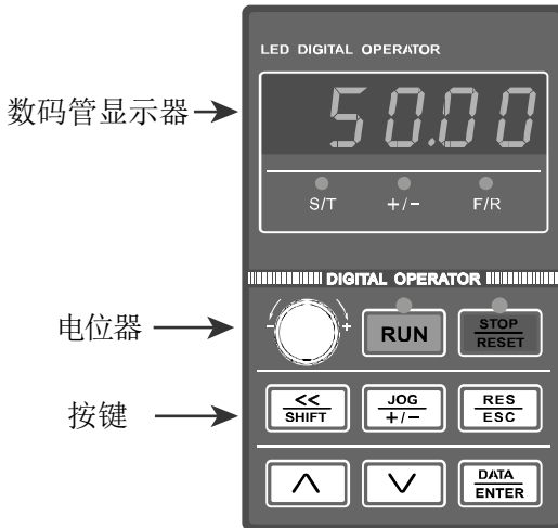
图 4-1 键盘各部件名称
