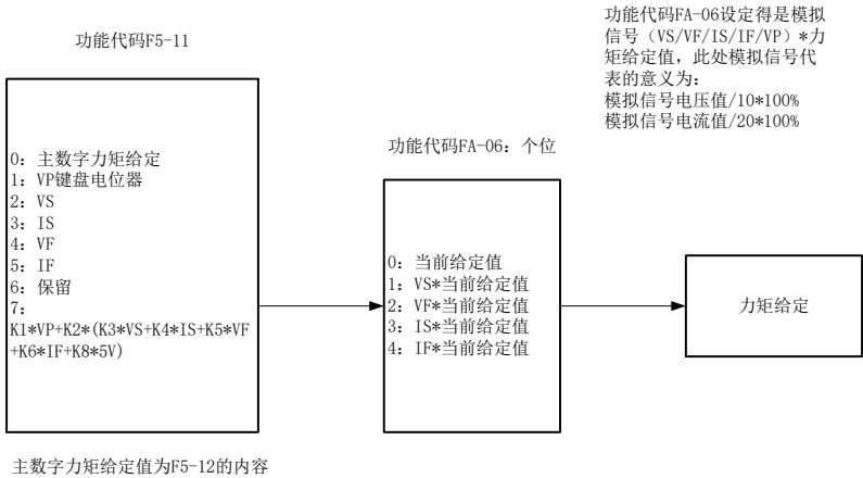
图 1-2 力矩给定方式示意图
