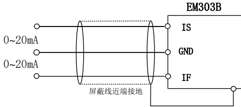
图 3-14IS、IF 端子配线图
