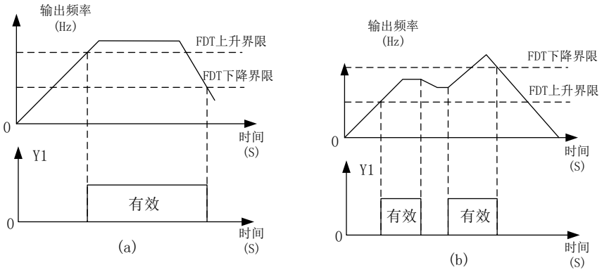
图 7-31 输出频率检测范围 FDT
