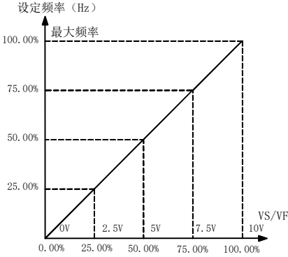
图 7-25 模拟电压输入 0~10V
