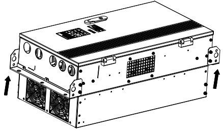
图 2-7 安装上下挂脚图示
