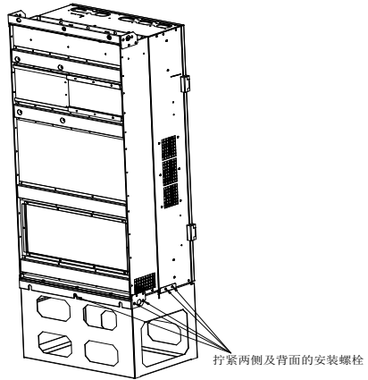
11-4 底座安裝图示
