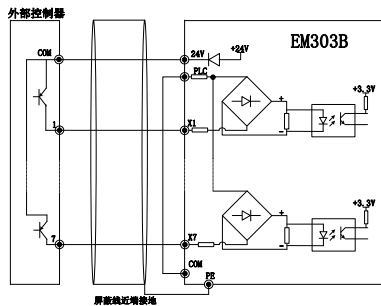
图 3-16 (b) 使用内部电源的漏极连接方式
