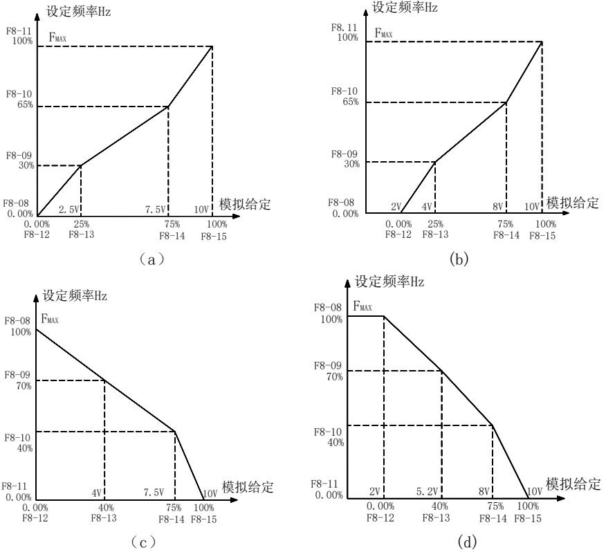
图 7-29 输入输出偏置
