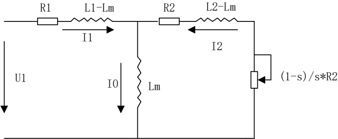
图 7-7 异步电动机稳态等效模型
