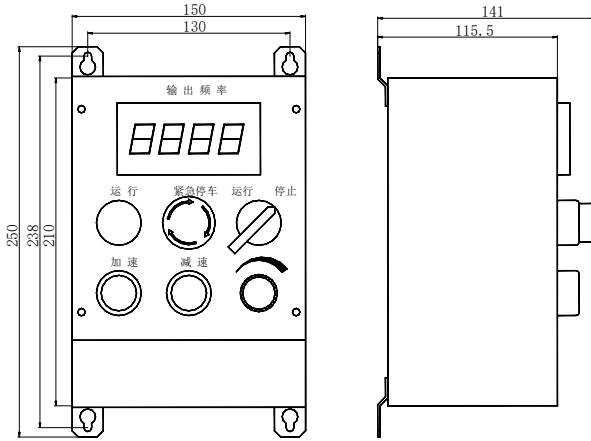
图 11-1 远程控制箱外形尺寸
