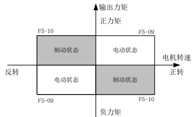
图 7-18 电动/制动力矩电流限定
