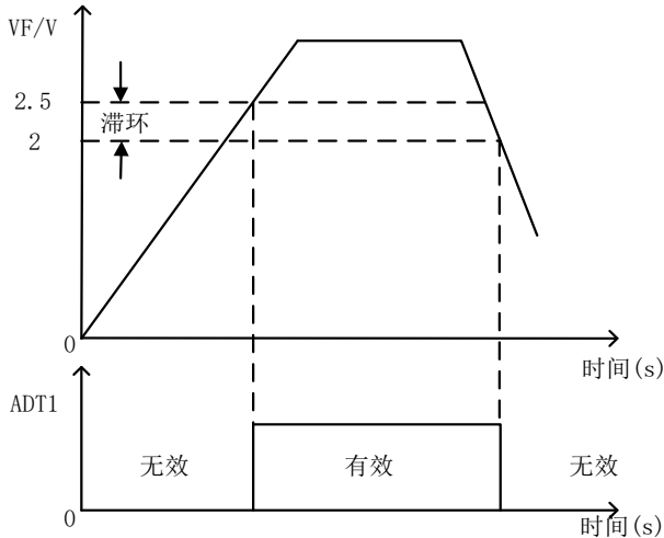
图 7-24ADT 功能示意图
