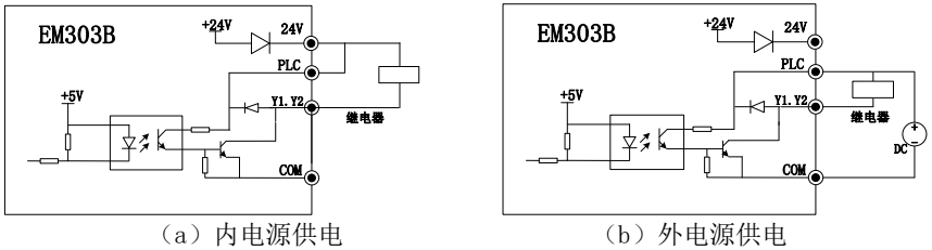
图 7-8 可编程端子供电方式
