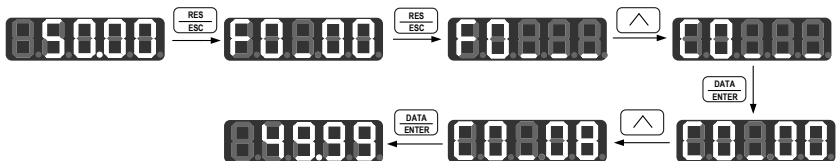
图 4-7 运行监视代码参数切换查询、修改操作流程
