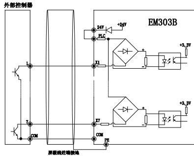
图 3-16 (a) 使用内部 24V 电源的源极连接方式
