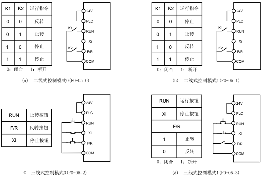
图 1-3 端子控制方式控制逻辑图
