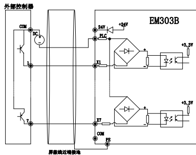
图 3-16 (d) 使用外部电源的漏极连接方式
