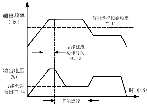
图 7-34 自动节能运行示意图
