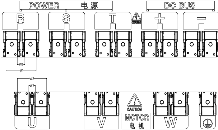
(d) 220kW-400kW 规格主回路端子
