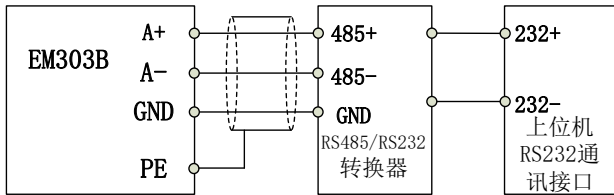
图 3-20 通讯端子配线
