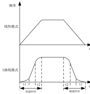
图 7-32 加减速时间控制图
