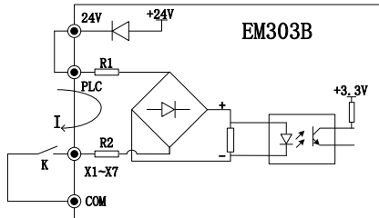
图 3-15 (a) 使用内部 24V 电源的连接方式
