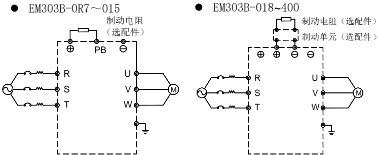
图 3-4 主回路标准接线
