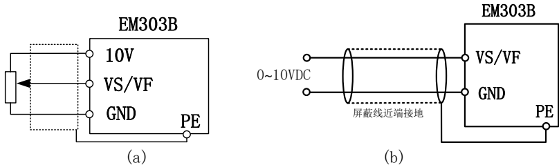
图 3-13VS、VF 端子配线图
