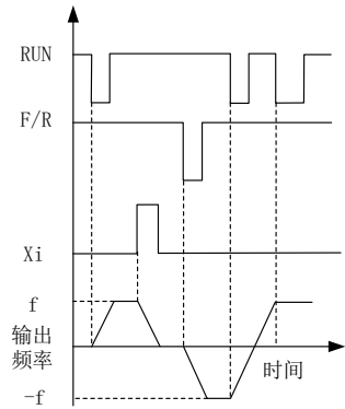
(b) F0-20=0, F0-05=2 正/反转运行逻辑
