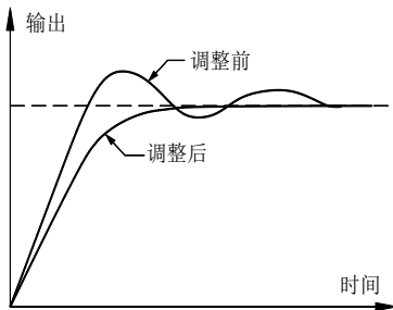
图 7-15 抑制输出超调图
