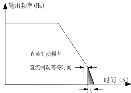
图 7-11 停车直流制动过程
