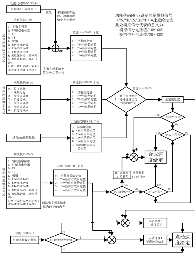
图 1-1 速度给定方式示意图
