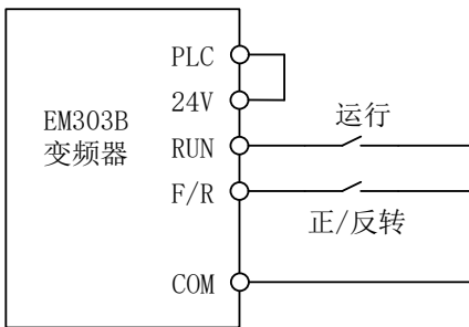
(a) F0-05=0 两线控制接线示意图
