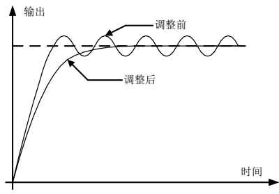
图 7-16 抑制输出周期振荡
