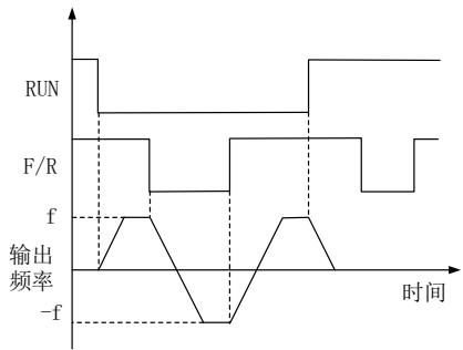
(b) F0-20=0, F0-05=0 正/反转运行逻辑
