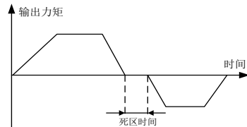
图 7-19 正/负力矩死区时间
