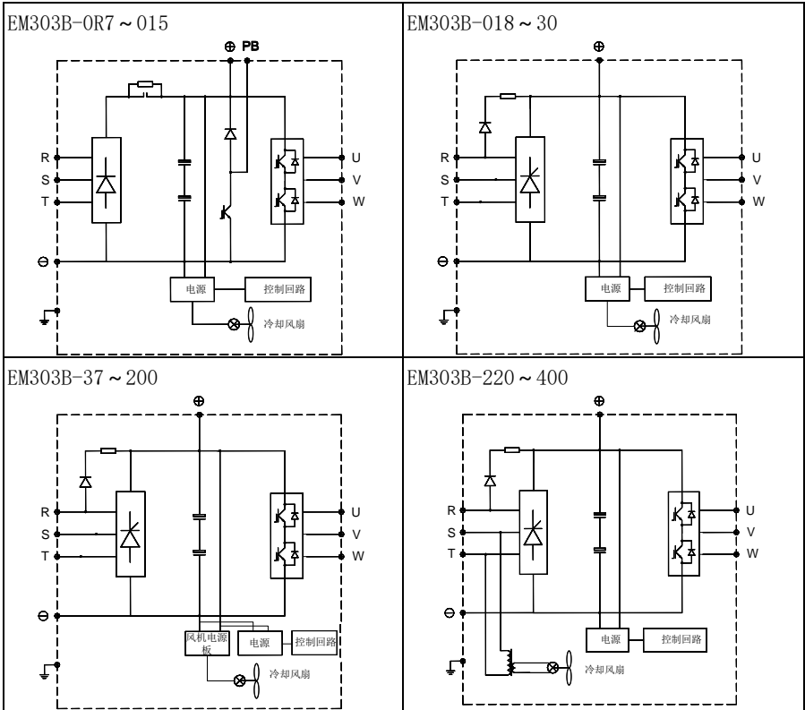
图 3-3 变频器内部主回路
