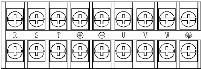
(b) 18.5~75kW 各规格主回路端子
