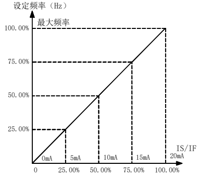
图 7-28 模拟电流输入 0~20mA
