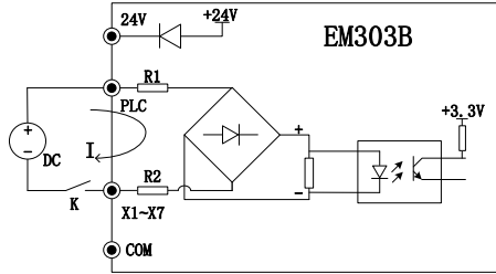
图 3-15 (b) 使用外部电源的连接方式
