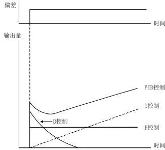
图 7-13PID 控制的作用
