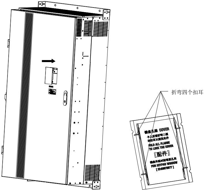
图 3-24 安装键盘孔盖板图示
