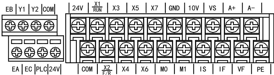
图 3-12 控制回路端子排列
