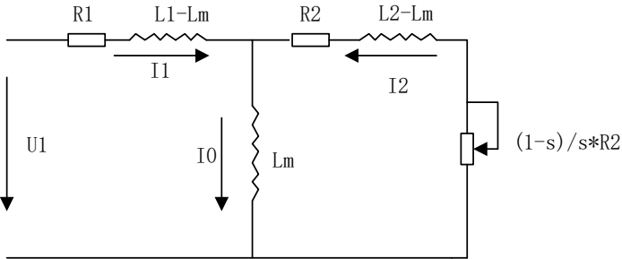
图 8-1 三相异步电机等效模型
