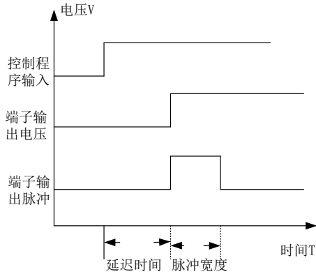
图 7-38 端子输出延迟时间
