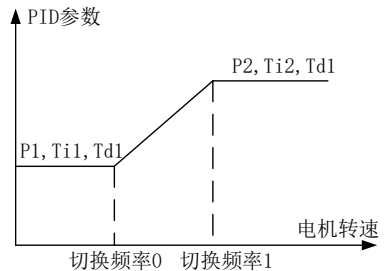
图 7-17 PID 参数示意图
