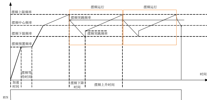
图 7-21 达到中点再摆频运行
