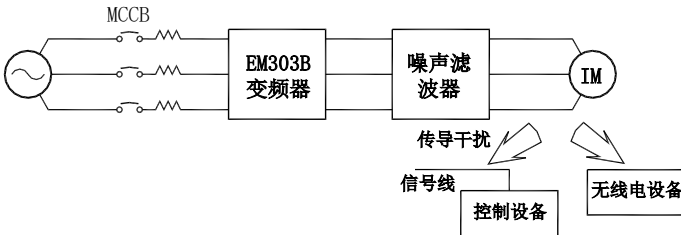
图 3-8 输出侧安装噪声滤波器
