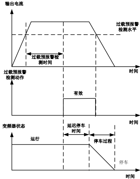
图 7-23 过载报警控制逻辑图
