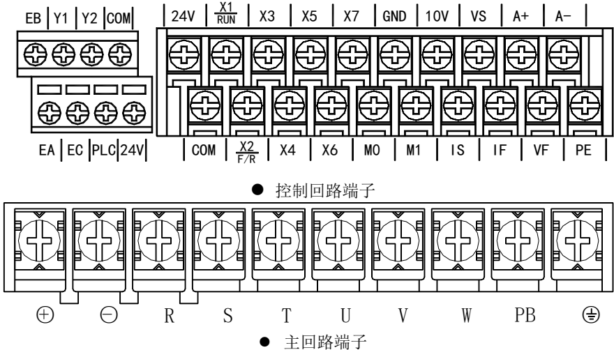
图 1-5 控制回路端子和主回路端子
