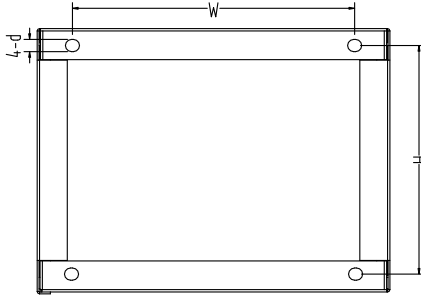
图 11-5 底座地脚螺栓安装孔尺寸图示
