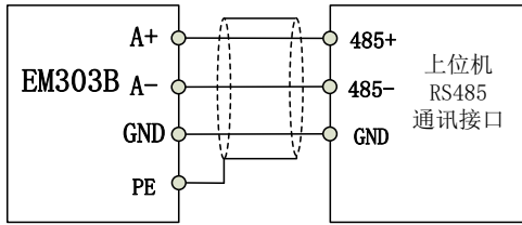
图 3-19 通讯端子配线
