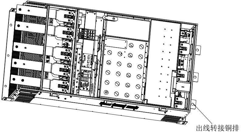
图 11-6 进出线转接铜排安装图示
