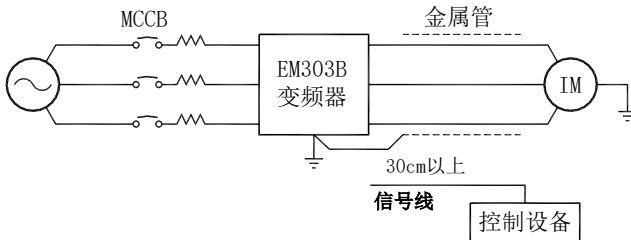
图 3-9 感应干扰对策
