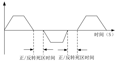
图 7-6 正/反转死区时间示意图
