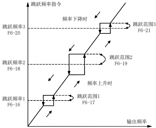
图 7-20 跳跃频率
