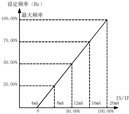
图 7-27 模拟电流输入 4~20mA
