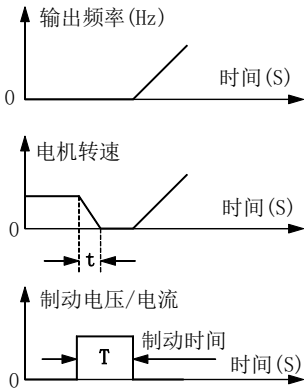
图 7-10 启动直流制动过程
