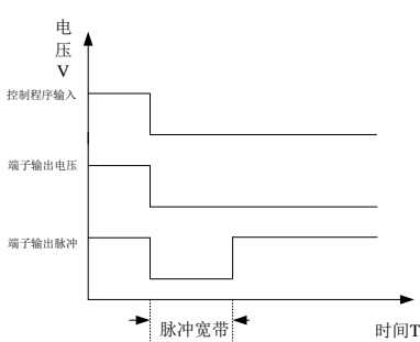
图 7-36 输出波形选择
