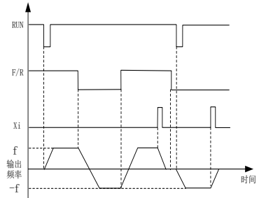
(d) F0-20=0, F0-05=3 正/反转运行逻辑
