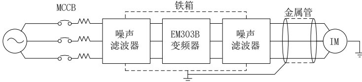
图 3-10 射频干扰对策
