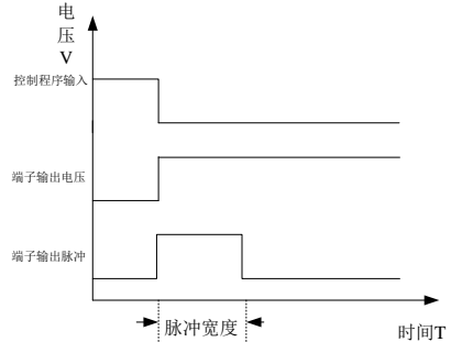
图 7-37 输出波形选择
