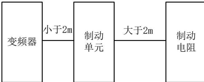
图 11-2 导线的长度
