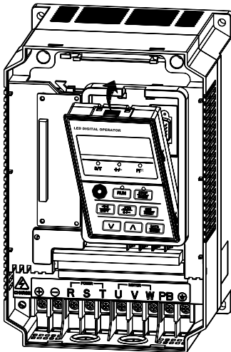
图 2-5 键盘安装图示
