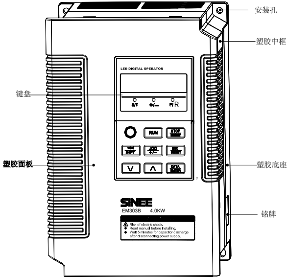
图 1-4 EM303B 系列变频器外型及部件
