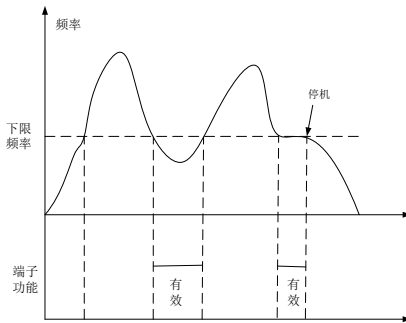
图 7-12 下限频率控制示意图
