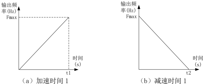
图 7-4 加减速时间
