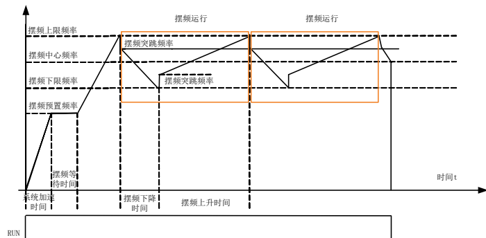
图 7-22 摆频预置时间到即开始摆频运行
