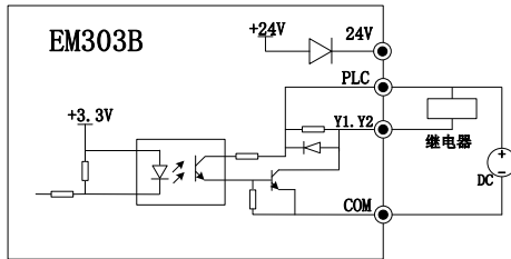
图 3-17 (b) 多功能输出端子用外部电源接线方式
