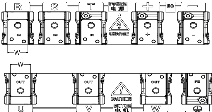
(c) 90kW~200kW 规格主回路端子
