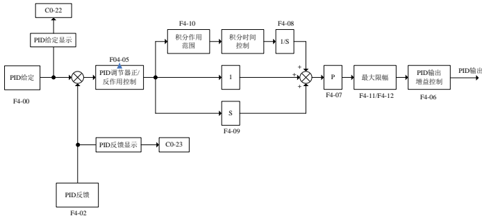
图 7-14EM303B 系列变频器内部过程 PID 的控制逻辑图
