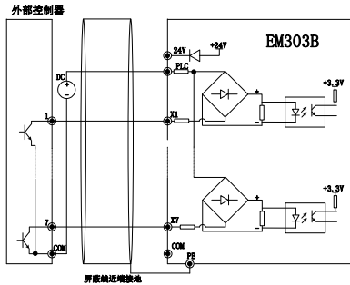
图 3-16 (c) 使用外部电源的源极连接方式
