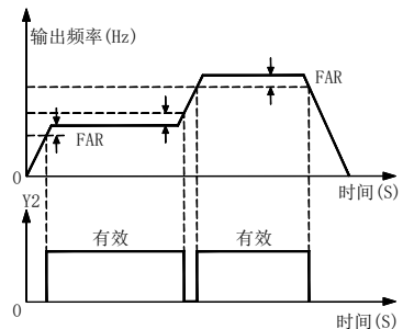
图 7-30 频率到达范围 FAR
