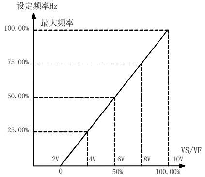
图 7-26 模拟电压输入 2~10V
